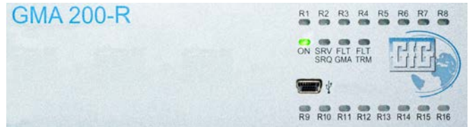
DEL d'état et port USB du GMA200-RT pour le GMA400
