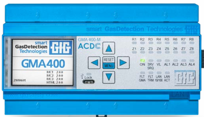
GMA400 - avec Modbus TCP et accès web via Ethernet
